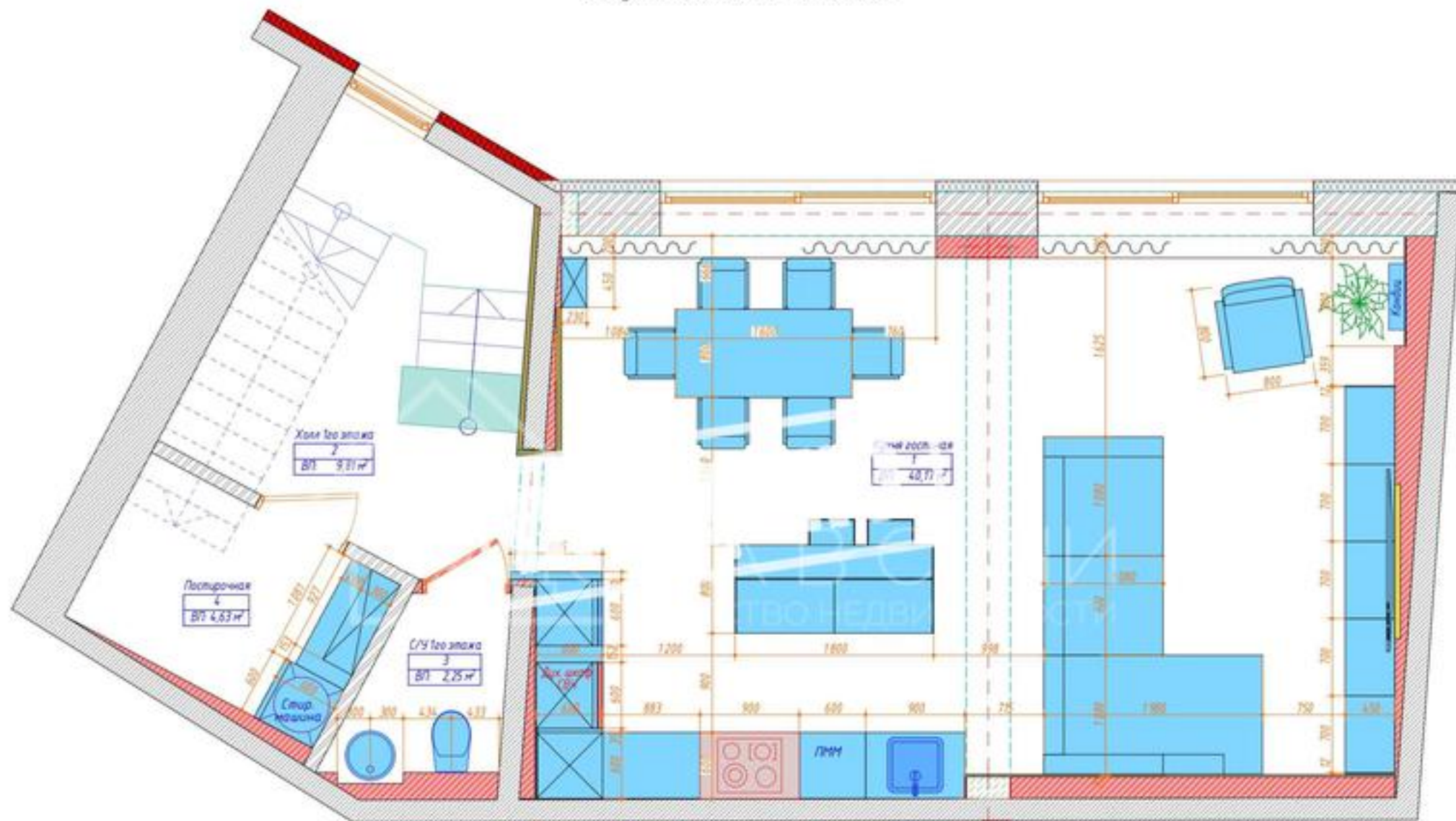
Экспликация 1-й этаж (Вновь возводим перегородок)
