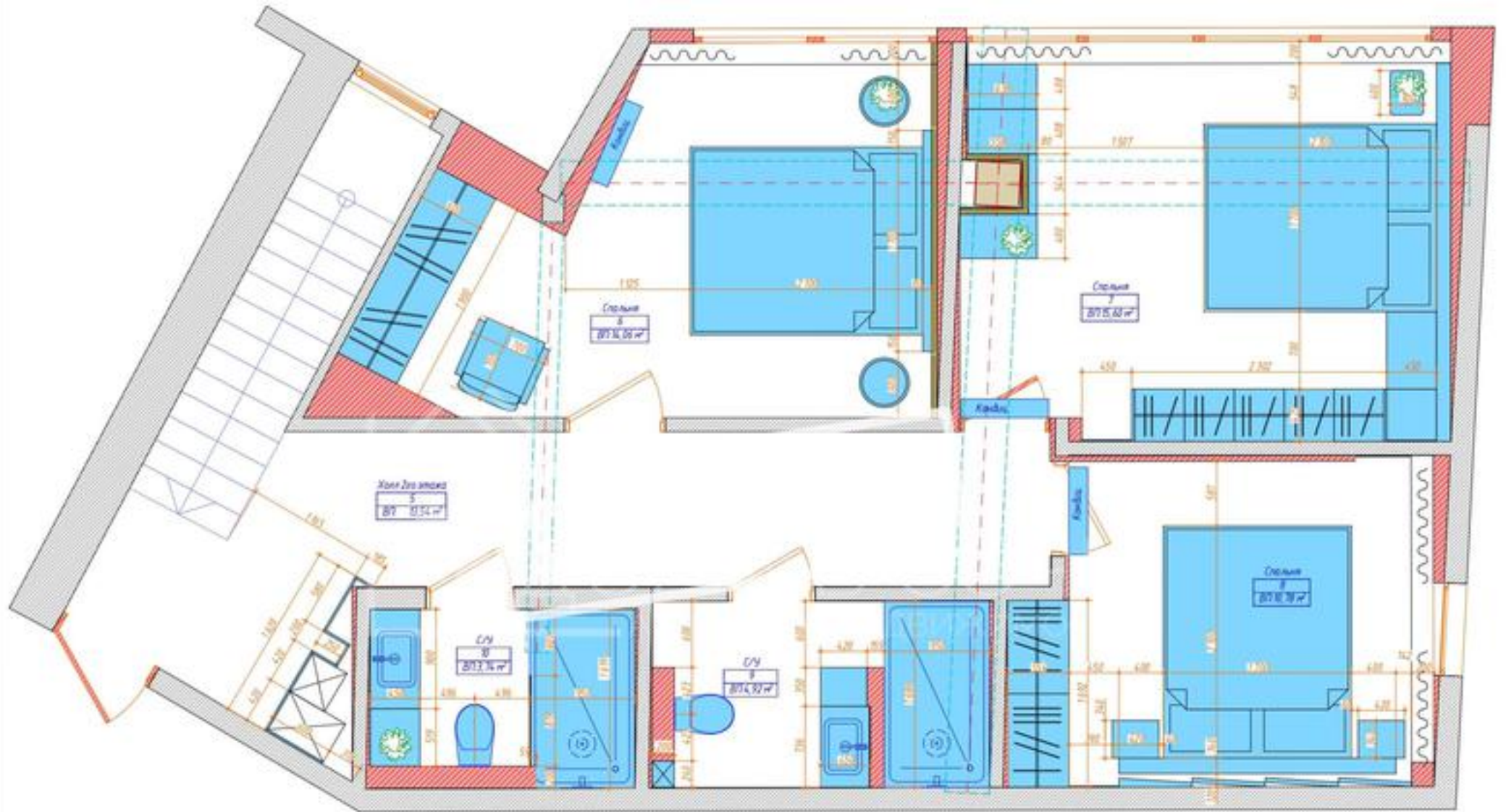
Экспликация 2го этажа (Вновь возводим перегородок)
